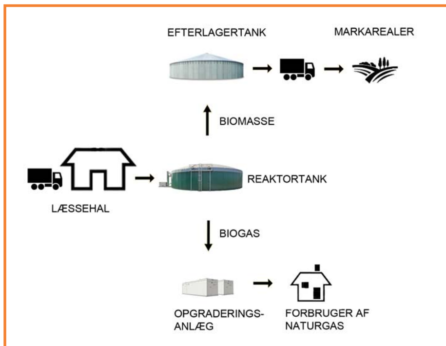
Flowdiagram – hovedprocesserne i Fuglsang Biogasanlæg
